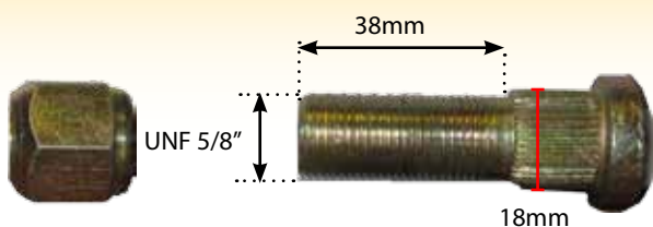
Trailer Hub Bolt 5 Stud
